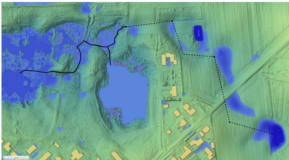
Figur 1: Analyse af oversvømmede områder ved 5 cm vand. Blå felter: oversvømmes i begge scenarier. Lilla felter: drænes hvis tørvegrøfterne udgraves (solid linje).
